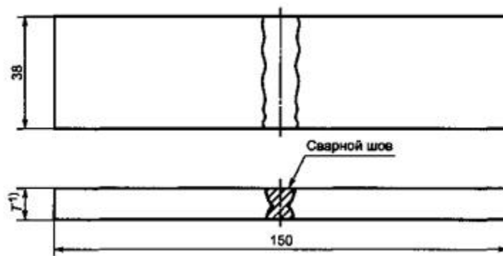
Рисунок 5 - Расположение образцов для испытания на ударный изгиб
