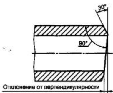
Рисунок 1 - Отклонение от перпендикулярности торца (косина реза)
