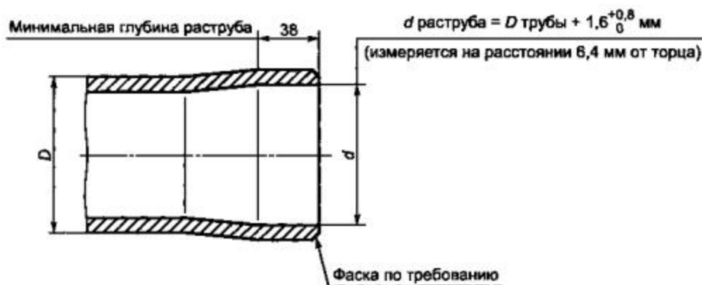
Рисунок 2 - Раструбный конец для соединения труб между собой
